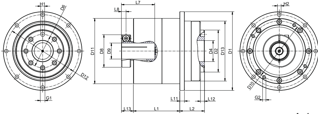
1-stage
